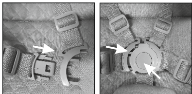
Пристегивание
